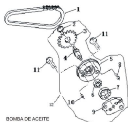
BOMBA DE ACEITE
